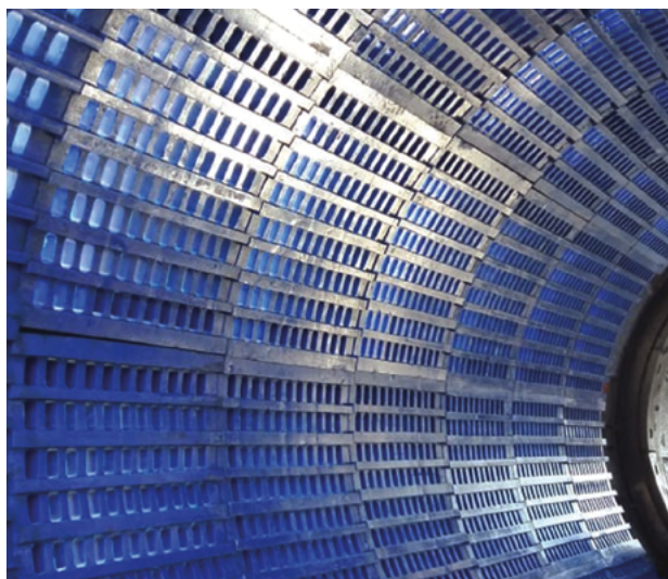
Instalación de las nuevas mallas de clasificación del trómel
